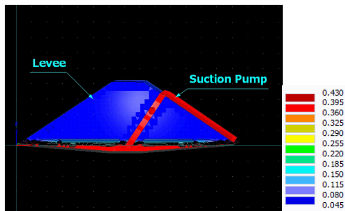
図 17 1 時間後の水分量（体積含水率）
