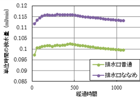
図 16 排水口形状・単位時間当たりの排水量
