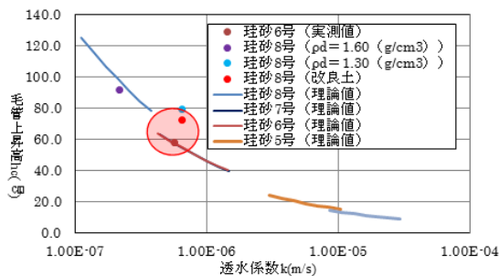
図 14 毛管上昇高と透水係数の関係
