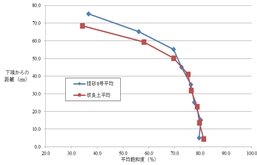
図8 平均飽和度の比較 (各4回の平均値)
