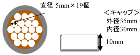
図4 アクリルパイプ断面
