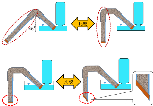
図5 各形状のサクシヨンポンプ
