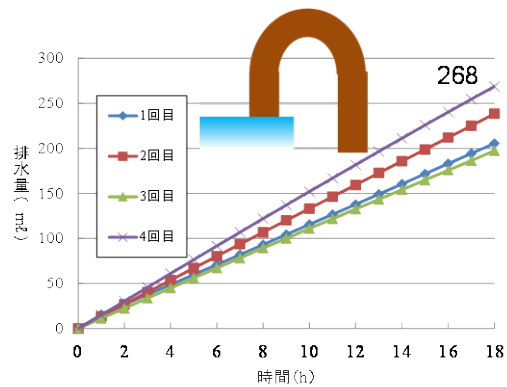
図10 繰り返し排水量の推移 (Case1)
