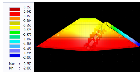
図7 初期条件(ポンプ断面)
