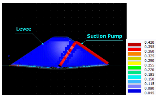
図 18 4 日後の水分量（体積含水率）
