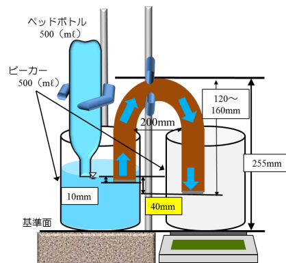
図3 サイフォン実験
