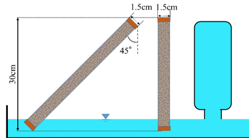
図2 形状による毛管上昇の検討
