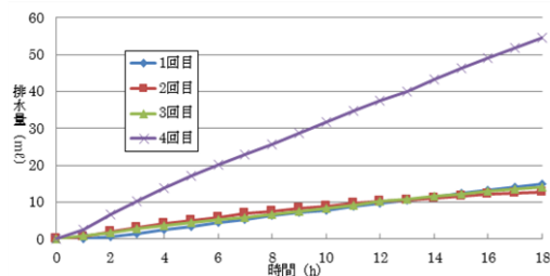
図12 繰り返し排水量の推移 (Case3)
