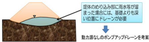
図1 堤体内の閉封飽和域と内部液状化
