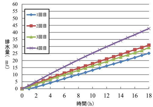
図11 繰り返し排水量の推移 (Case2)
